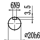
输入轴
