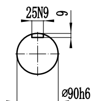
入出力轴
