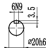
输入轴
